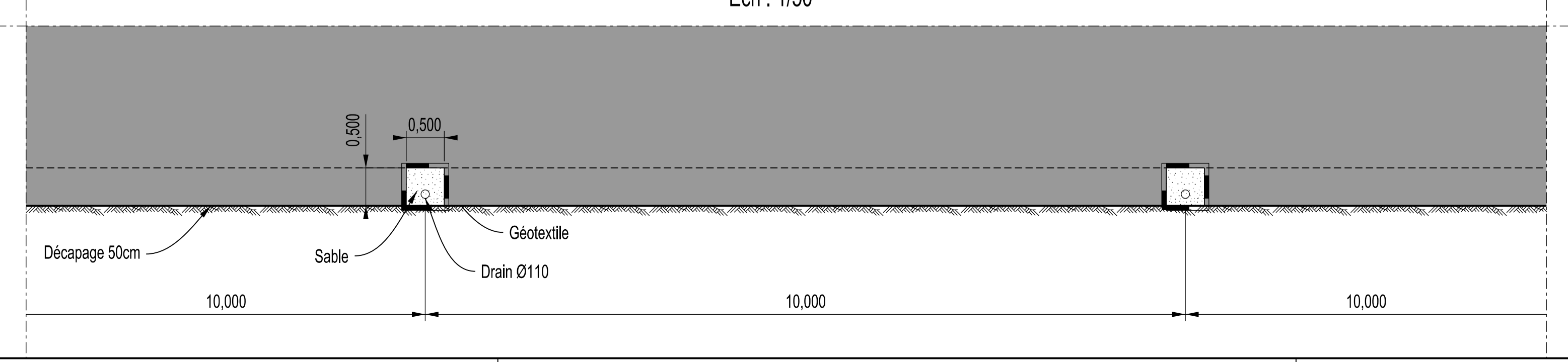
DETAIL C Ech : 1/50
